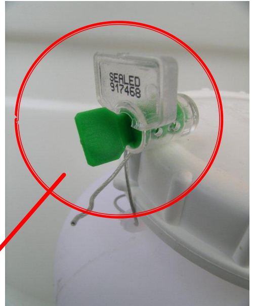
BOTELLA : PL 33 Capacidad litros : 4 Lt Altura : 29,5 cm Diametro: : 15,5cm Boca diam : 8,2 cm
